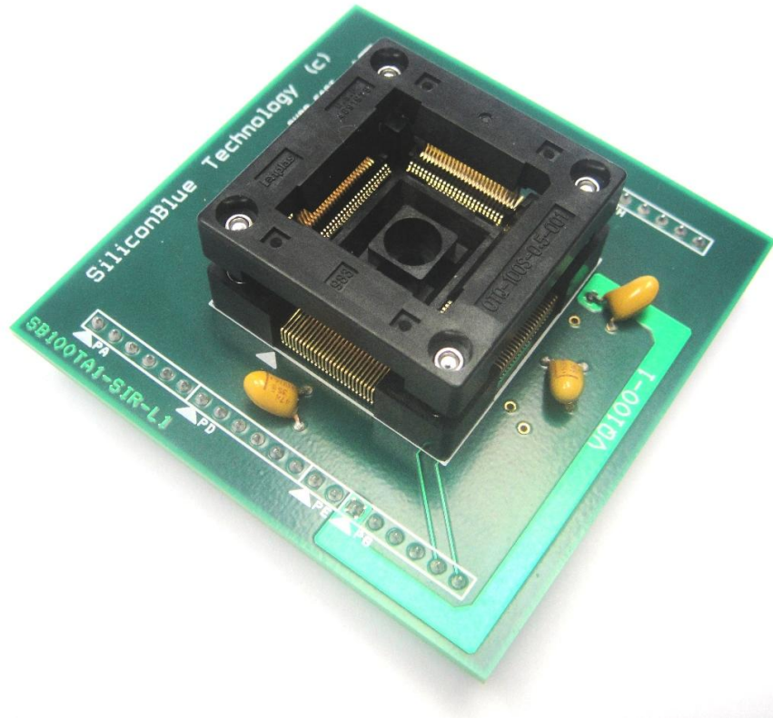
Figure 1: iCEsabVQ100-01
